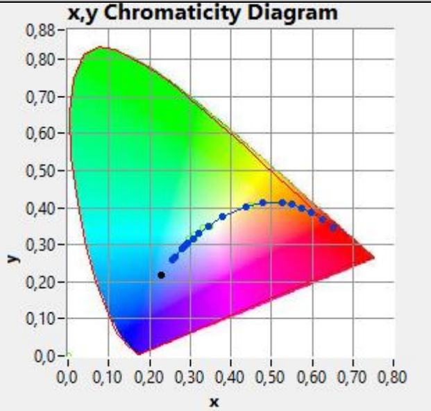
GRÁFICO CIE 1931
