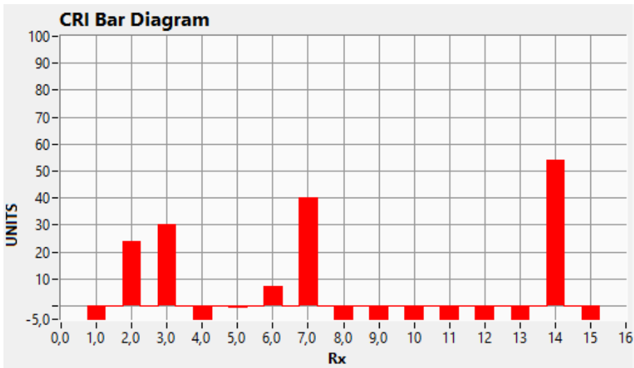
DIAGRAMA CRI
